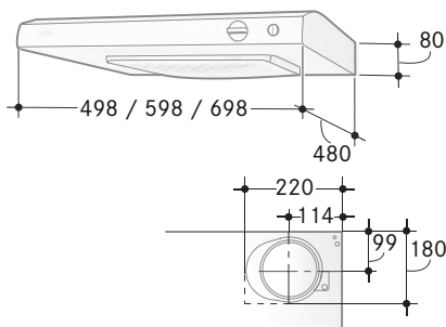
Spisfläkt 210, 210 Safe, 215
