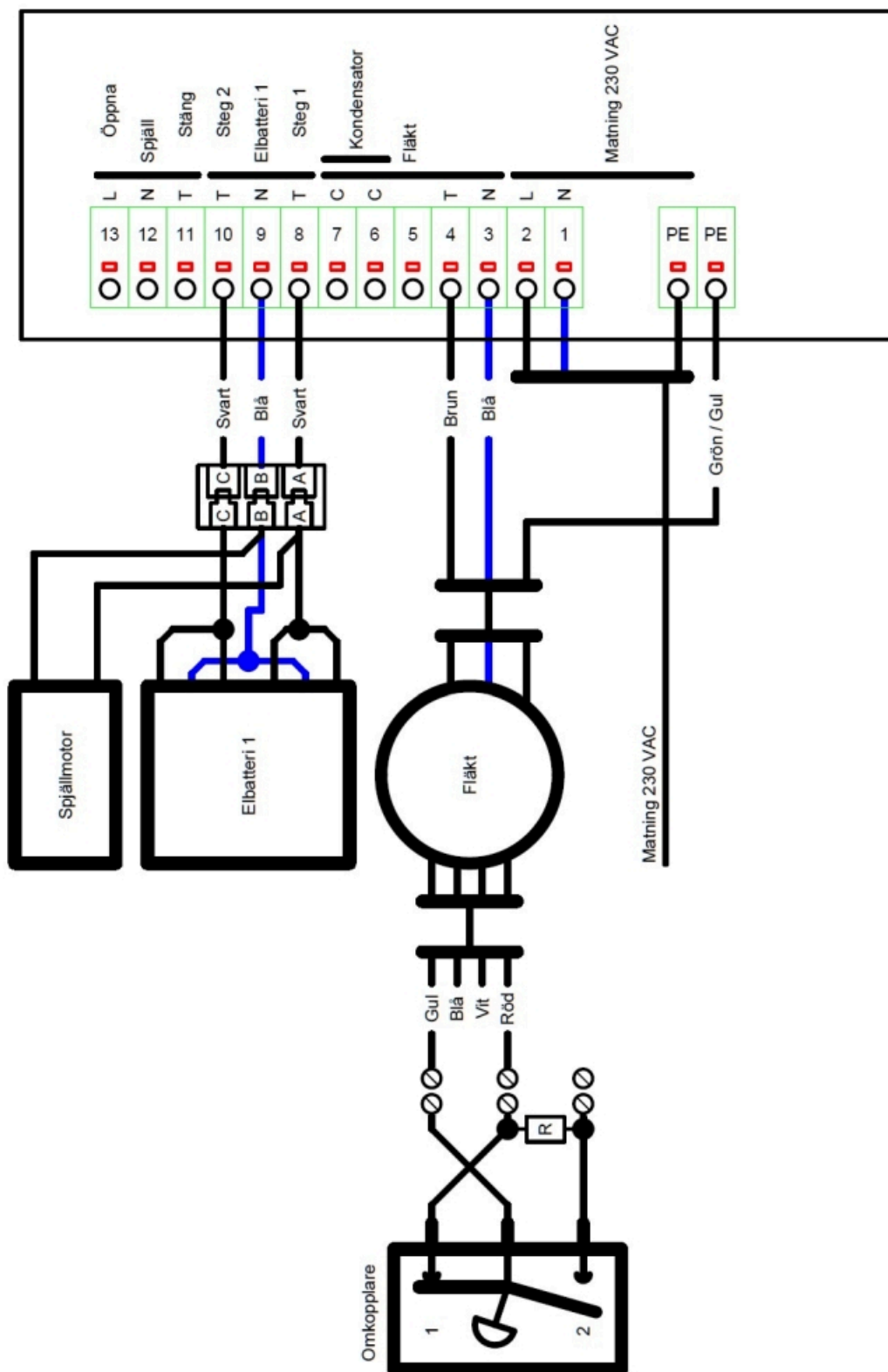
Eischema RD
