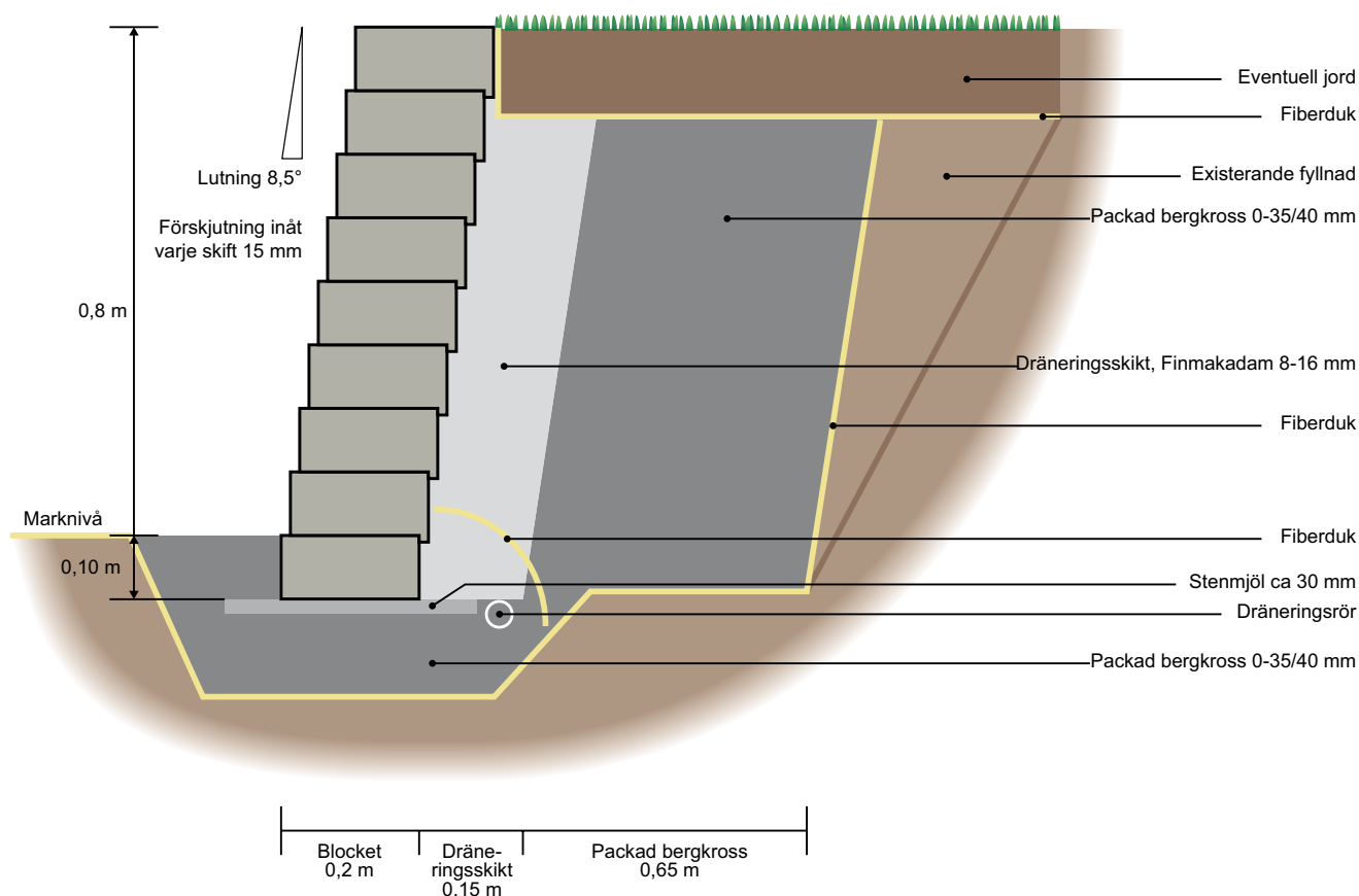
Bild 1. Sektionsritning Megastone Mini Rakhuggen 300 x 200 x 100.
