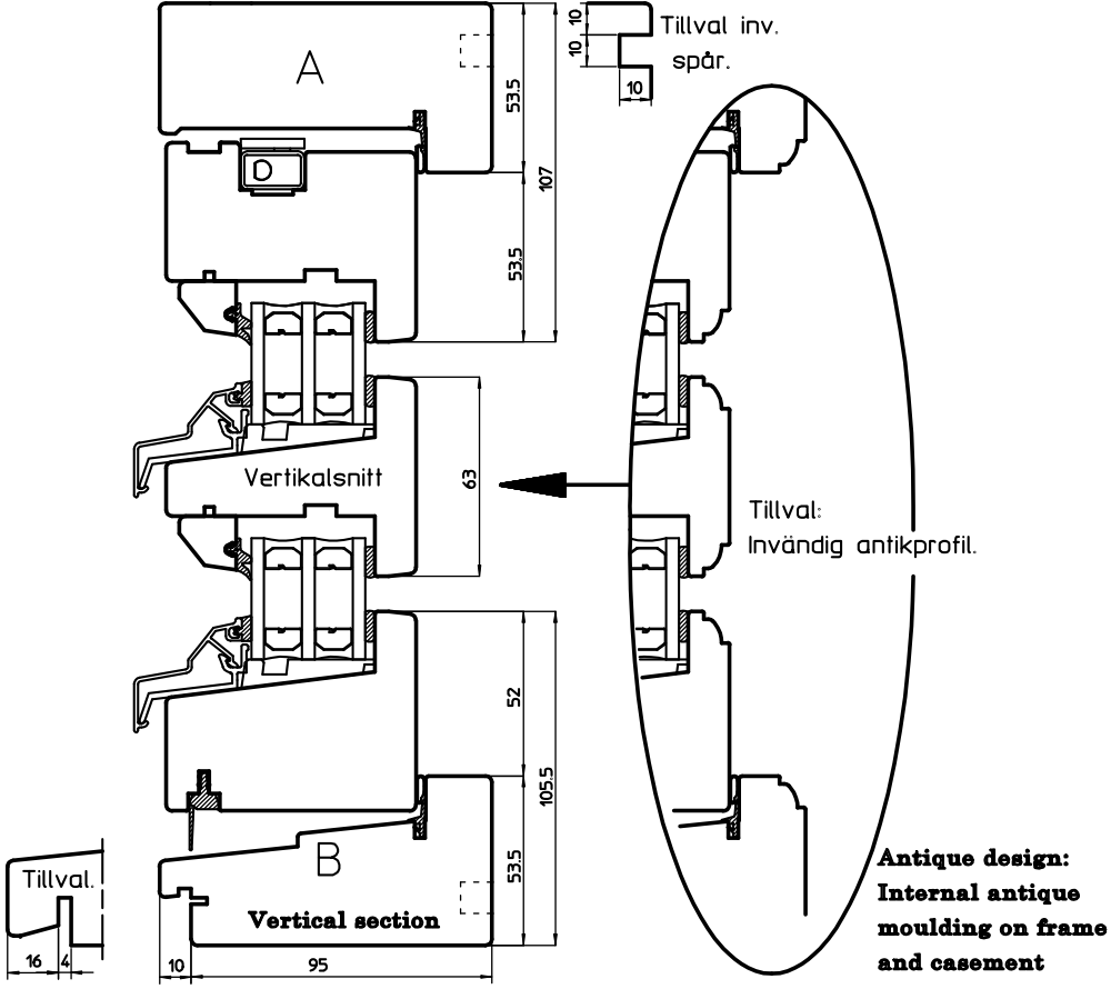
Kombination, vertikalsnitt sidhängt+ glidhängt på höjden
