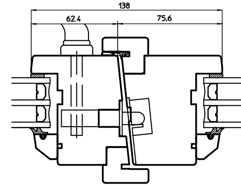
Horizontalsnitt mötesbåge Horizontal section abutting casements
