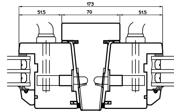
Horizontalsnitt 2-luft Horizontal section 2 lights
