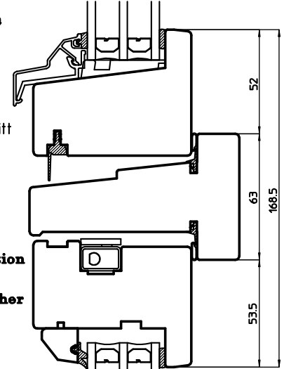
Horizontalsnitt 2-luft Horizontal section 2 lights
