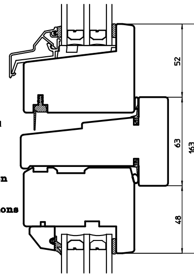
Horizontalsnitt mötesbåge Horizontal section abutting casements
